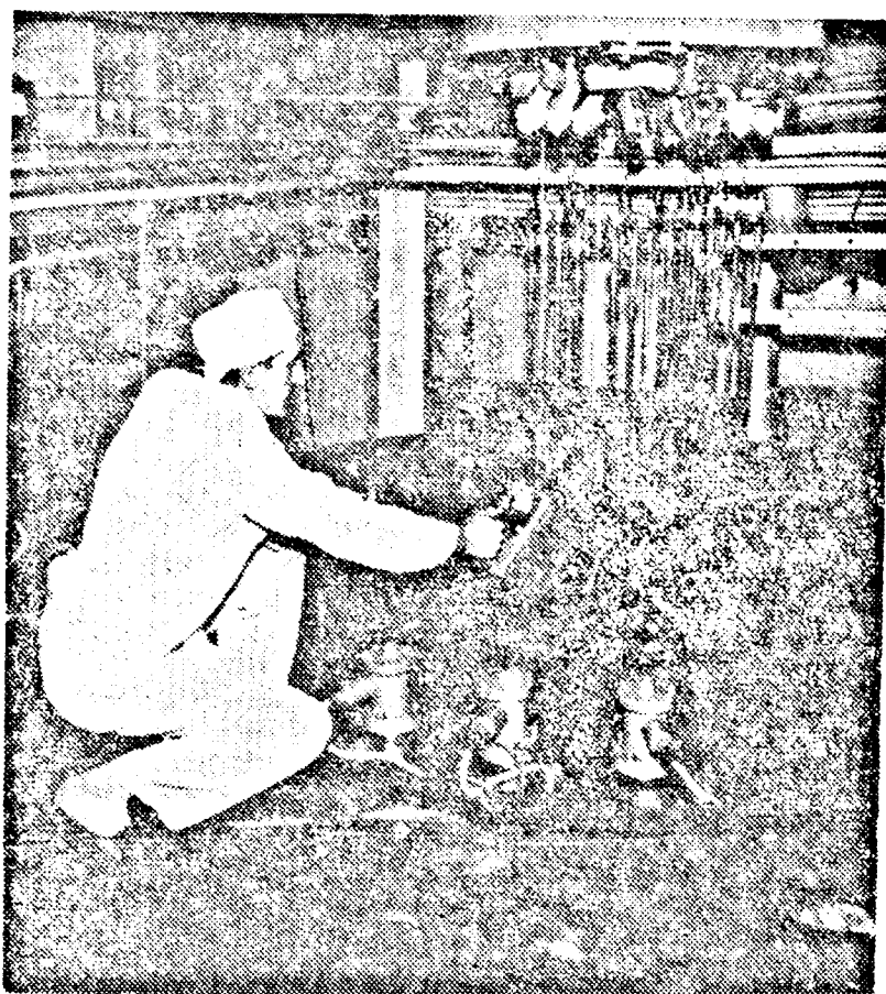
A szovjet szakemberek bordonható atomelektronikus központot készítenek. A központ szerkezetét különböző blokkok képezik, amelyeknek súlya darabonként 12-15 tonnát tehet. Az ilyen atomelektronikus központ termelési kapacitása 750 kilowatt energia. Képeknél: a berendezés sugárhatását ellenőrzik.
