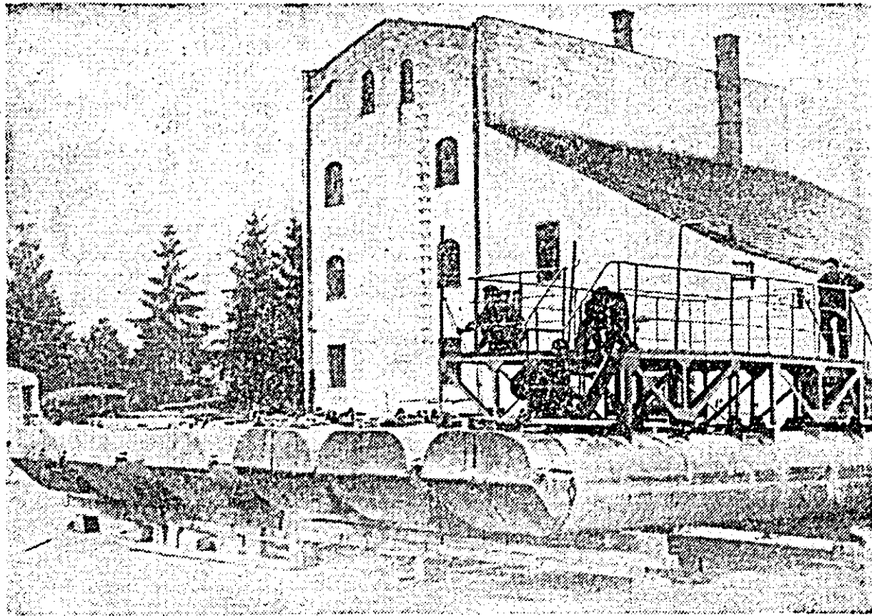
Cliseul nostru reprezintă 6 corpuri plutitoare din care vor fi asamblate 3 flotoare cu vinci și o platformă cu balustrade. Flotoarele cu vinci se numără printre produsele noi ale I.R. „Mureșul” din orașul nostru.
