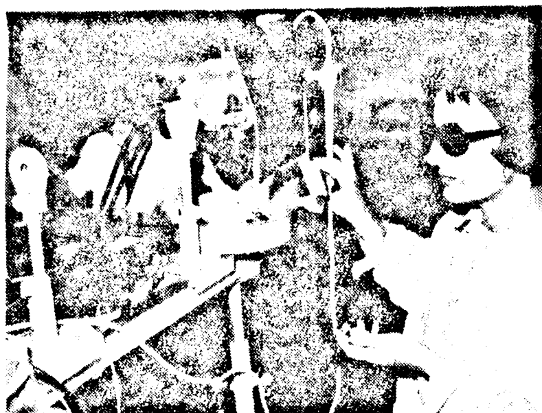
A fővárosi Geológiai Felülvizsgáló Vállalat spektrográfiai laboratóriumában kőzetek vizsgálata folyik.
