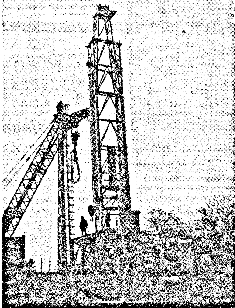
A ploiești-i I. Mai kőolajipari berendezéseket előállító üzem egyik újabb terméke, amely tíz különböző művelet elvégzésére alkalmas és 6500 méter mélységig képes fúrni.
