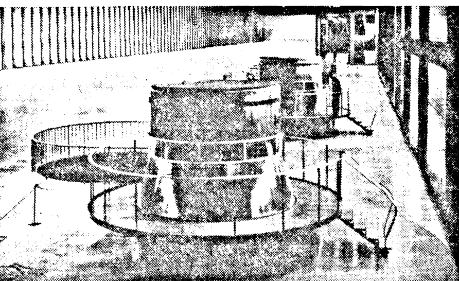
JUGOSZLAVIA SZSK. Képünk a Spili-vizi-erőmű gépteremében készült a hatalmas generátorokról, melyeket a zágábi „Rade Koncar” üzemben gyártanak.
