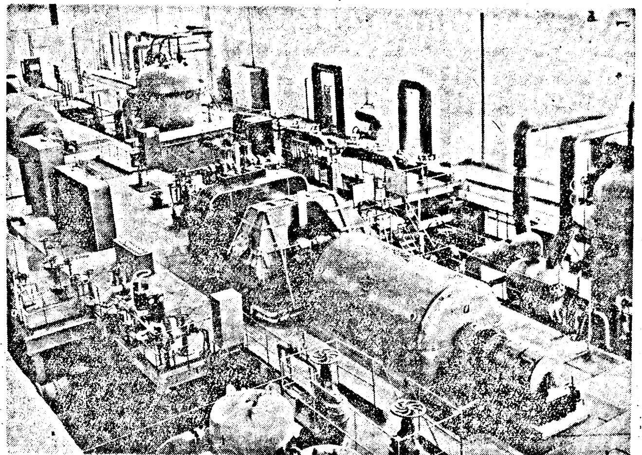
A borzești hőerőműben megkezdtek a harmadik 25 megawattos turbogenerátor, valamint a nagynyomású gőzturbinák felszerelését. A következő évek során a borzești hőerőmű villamos energia termelését 75 megawattal 125 megawattal emelik. A jövő év elején megkezdik az első 50 megawattos turbogenerátor szerelését.
