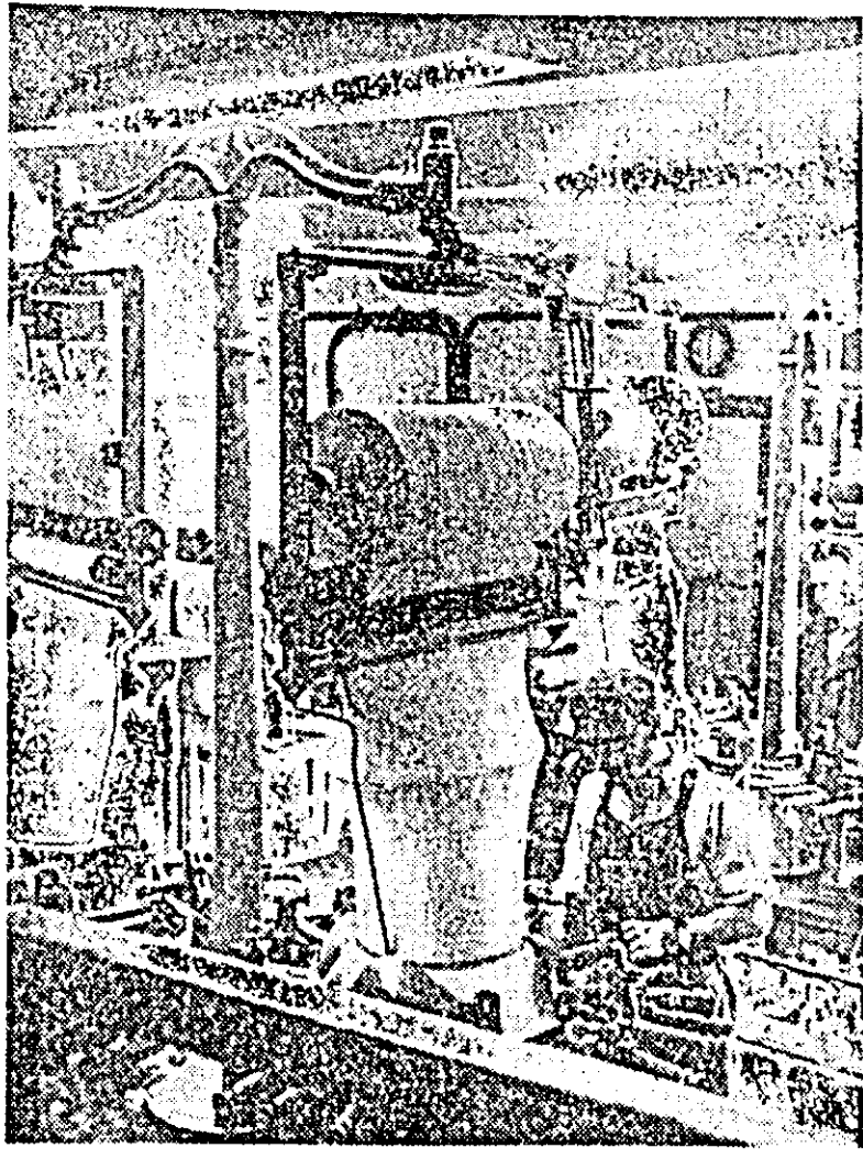
Aspect din secția de tricotat circular a fabricii „Tricoul roșu”.
