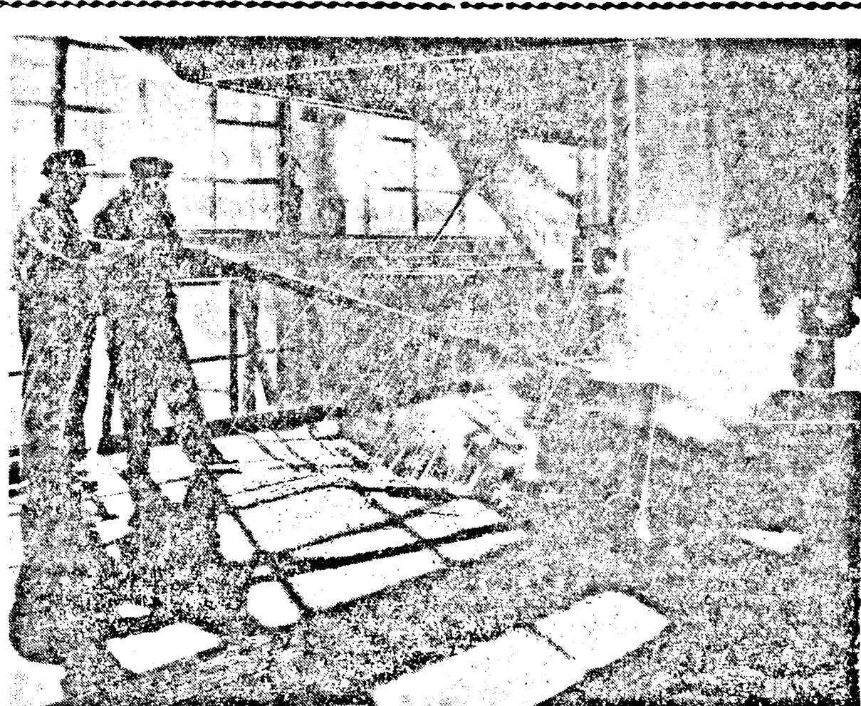
A kolozsvári Carbochim ipari méreteiben gyártja a csiszolókövek egyik fontos alapanyagát, amelyet még nemrégiben magas áron külföldről kellett behozni. Felvételünk az egyik nagykapacitású villamoskemencéről készült.
