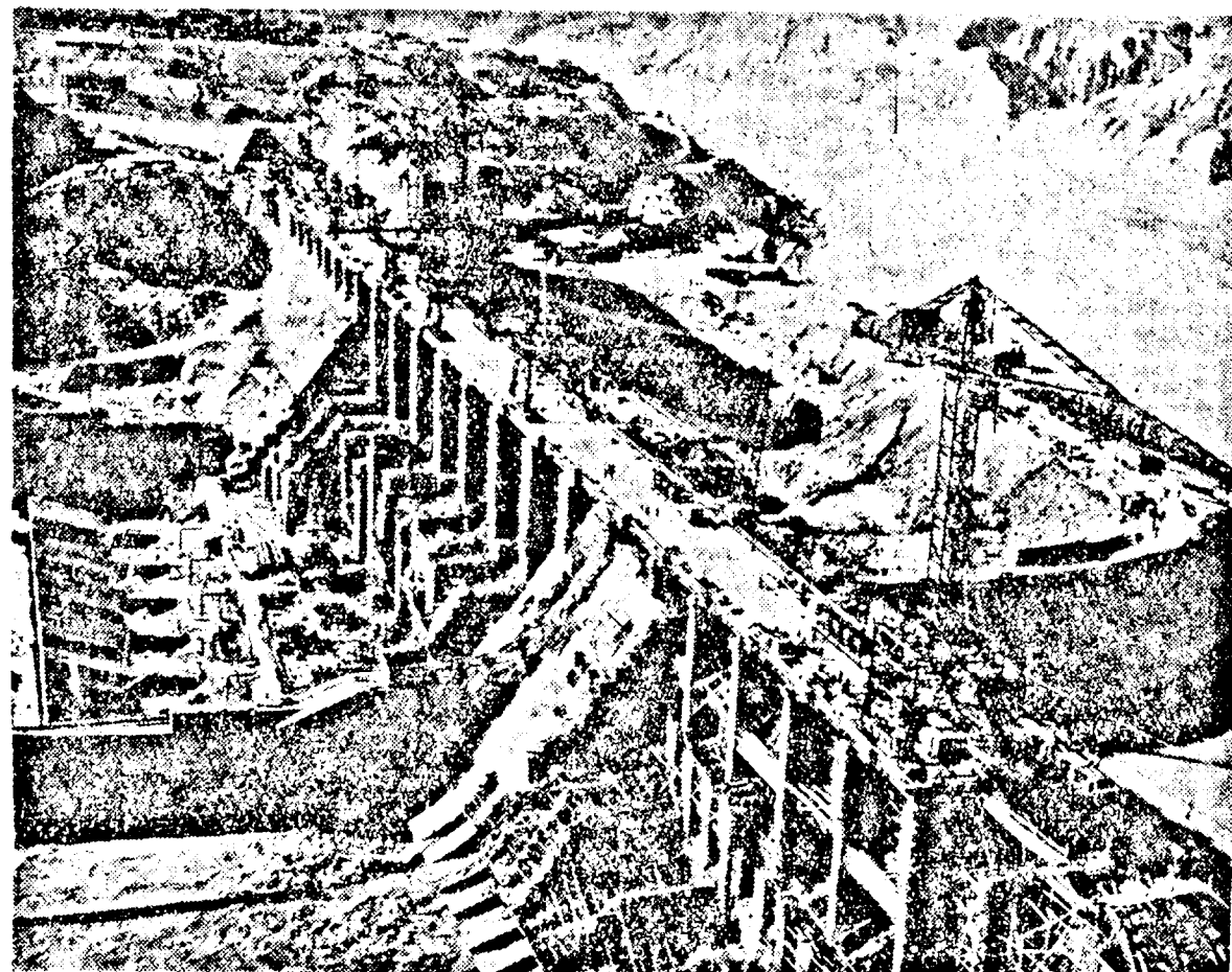
A Honan tartományi Szan-Men folyó torkolatánál történő vízellátási munkálatok lehetővé teszik majd az áradások szabályozását. Mult év december 9-ig teljesítették az 1959. évi tervtervadatot: 1 millió tonna vasbetont öntöttek, a felhasználott vasszerkezet összesen 6500 tonnát tesz ki. A munka minősége elsőrangú s ugyanakkor jelentősen csökkentették az előállítási költségeket. Képek: gyors ütemben végzik a földzáró gáton a vasbetonöntést és a fém szerkezeti részek szerelését.
