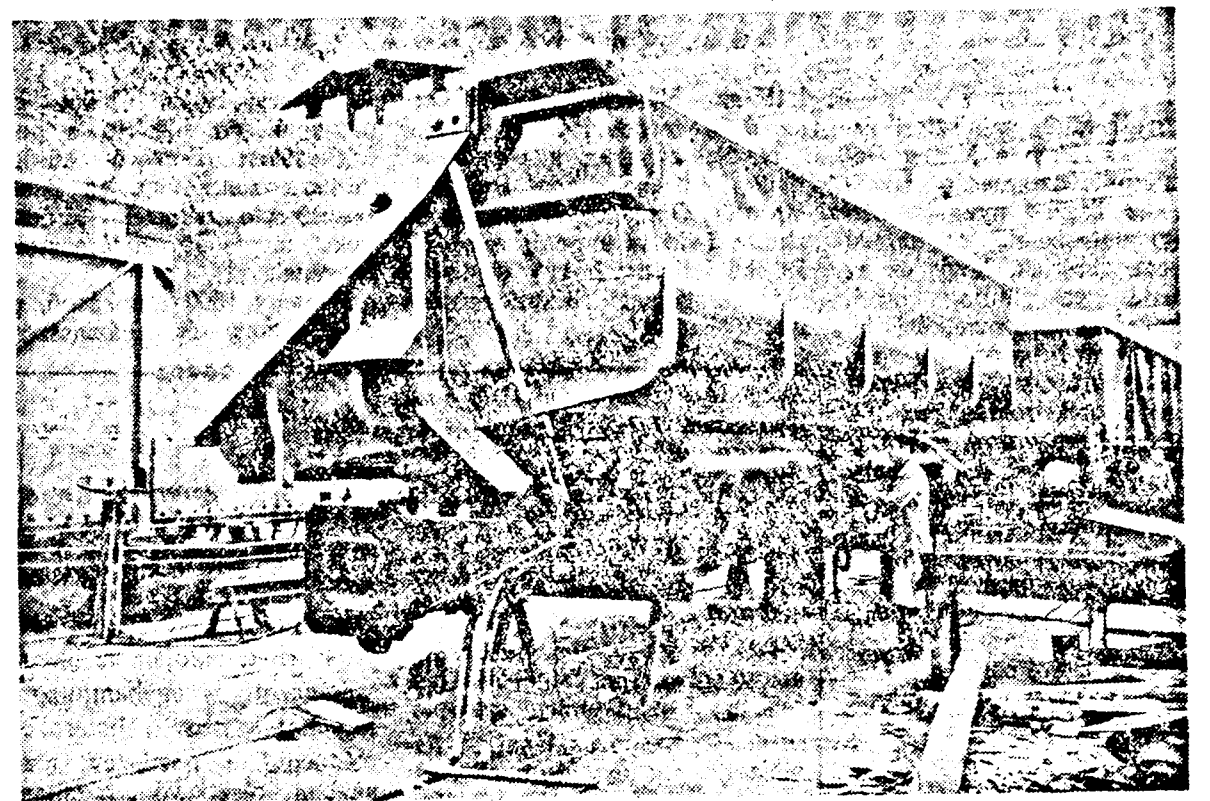
A Dimitrov-gyárban megkezdtek a 40 köbméter űrtartalmú 80 tonnás billenő vagonok sorozatgyártását. A golyós csapágyon forgó négy tengelyes vagonokat automata fékekkel látták el. A sűrített levegővel működő billenő szerkezet segítségével a vagon néhány perc alatt kiüríthető. Képünkön a billenő vagon látható szerelés közben.
