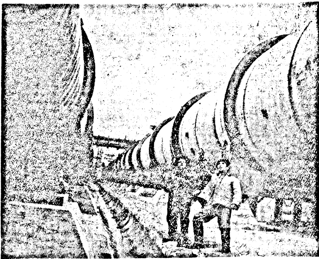
A Stejaru-i villanygyárban Popa Gheorghe és Cofocar Vasile szerelők a hatalmas csővezeték befejezési munkálataira készülnek
