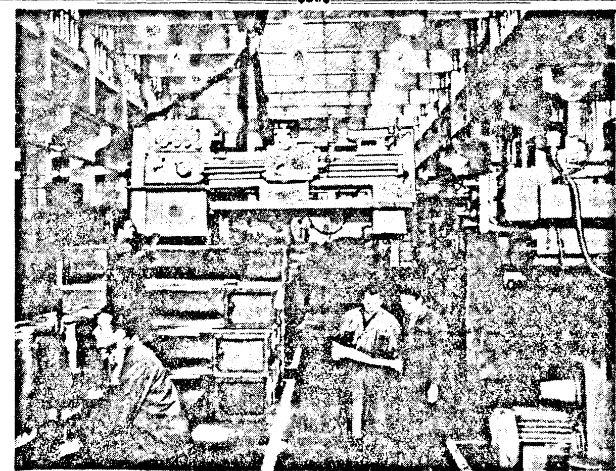
Ismét elkészült egy esztergagép a Ranghet szerszámgépgyárban. Az előtérben Rosenfeld Pál előrajzoló, a háttérben Sümei József főmester és Hermle István váltómester egy rajtot tanulmányoznak. A daru pedig, mint engedelmes óriás viszi az új esztergagépet a „szállítópályára”. Kész, mehet.
