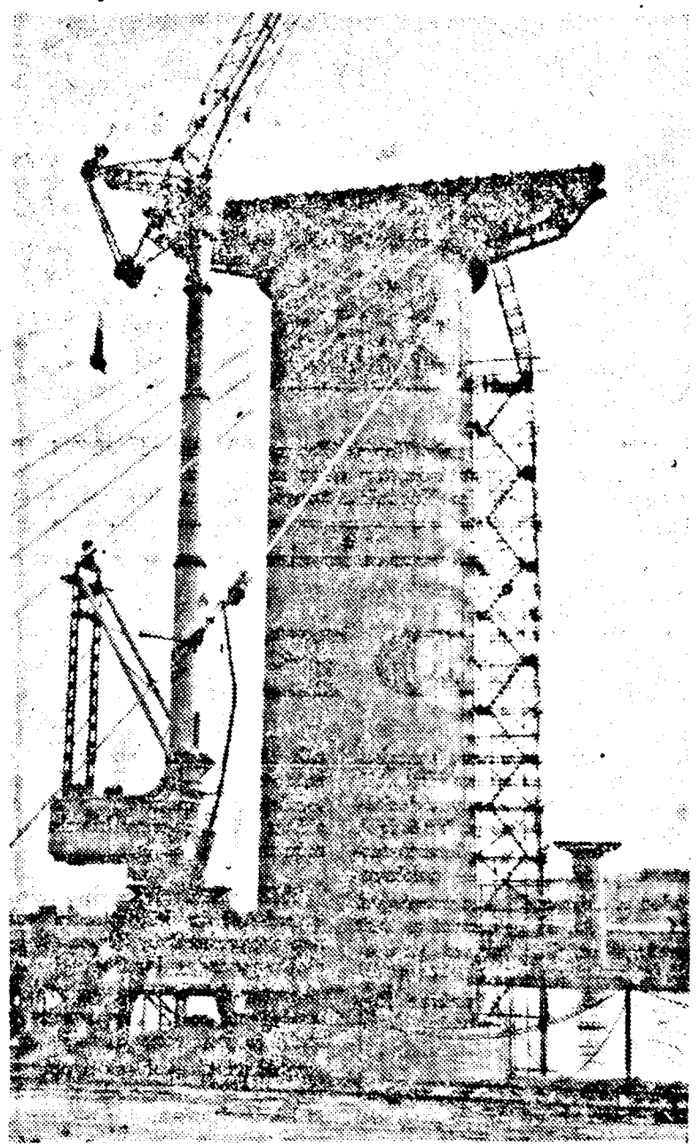
A Vankapu építőtelepe... A Dunát átszelő anyagszállító drótkötélpálya egyik „lába”.
