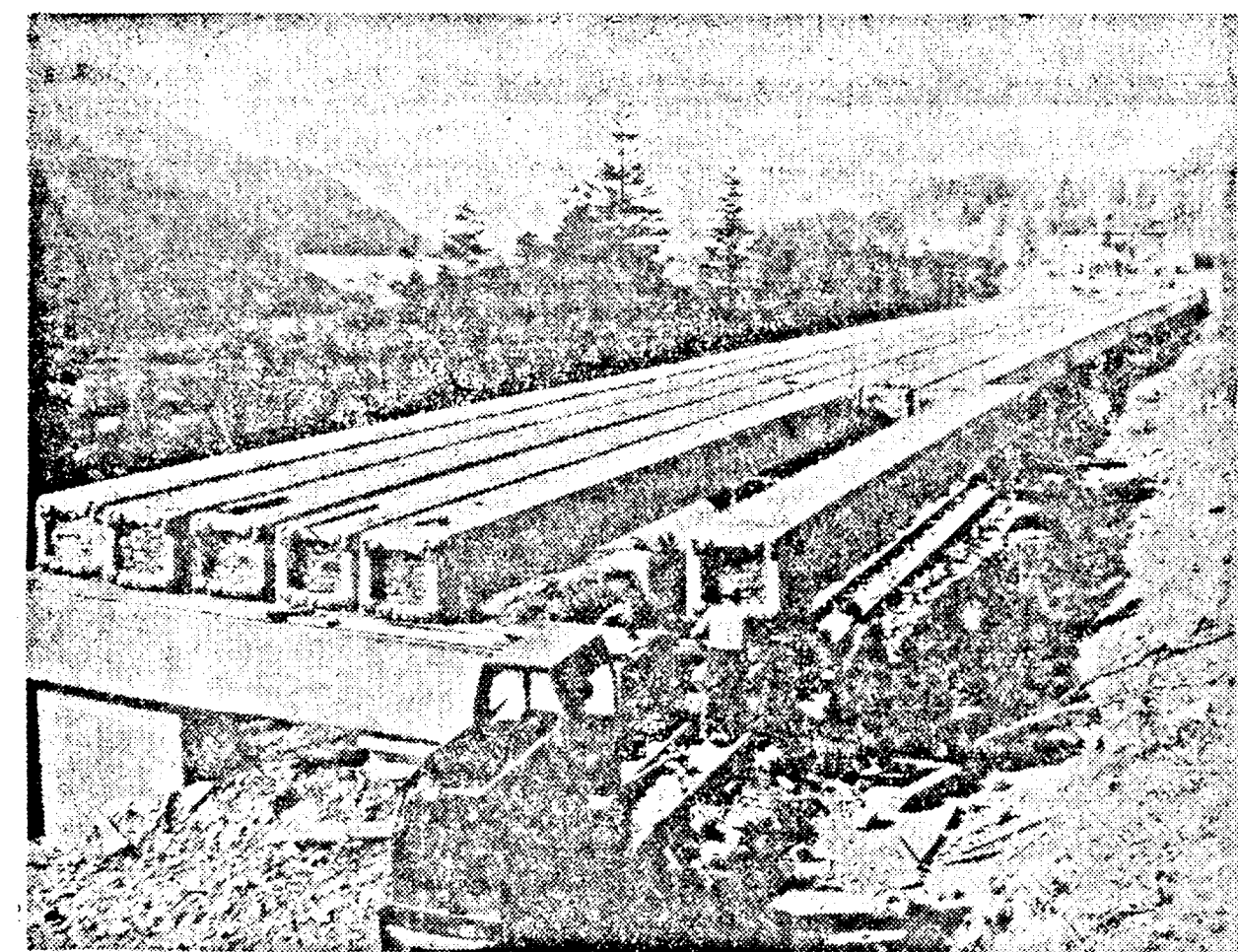
CSEHSZLOVÁK SZOCIALISTA KÖZTÁRSASÁG. Megkezdtek a betonalapozási munkát a Vltava folyón építendő hatalmas hídhoz.
