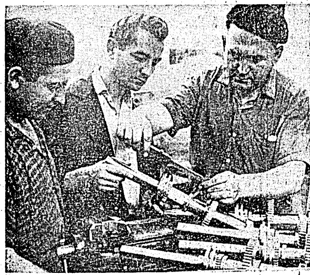
Colectivul secției montaj-parțial de la Uzina de strunguri acordă toată atenția calității produselor. În cliseu: montatorul Carol Benke, maestrul Petru Strimle și controlorul de calitate Alexandru Alieș, verificînd un nou lot la axele principale ale strungului SN 250.
