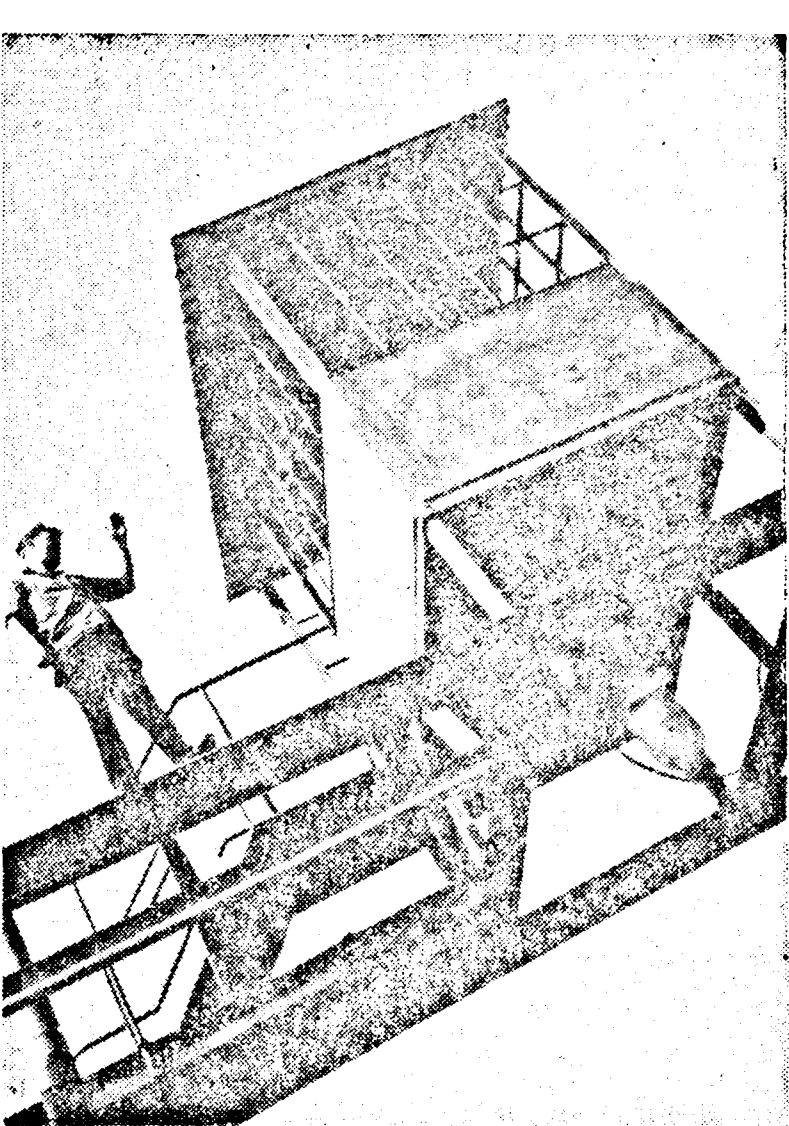
Nemrég helyezték üzembe az aradi Cukorgyárban a képkönn látható berendezést, mely vizsugar segítségével üríti ki a cukorrépat a vagonokból.
