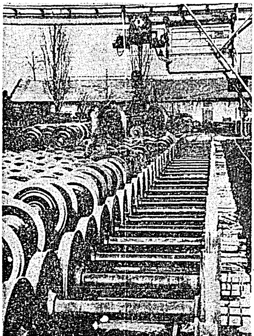
Aspect al depozitului de roți de la Uzinele de vagoane.
