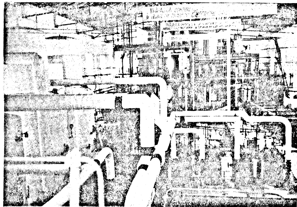
Képünkön az aradi Cukorgyár főző részlegének „megfiatalított” gépei, kazánjai és csőlabirintusa látható. Baloldalt a vákummal dolgozó kazánok, melyek az új idényben már eddig is több tonna jó minőségű cukrot főztek.
