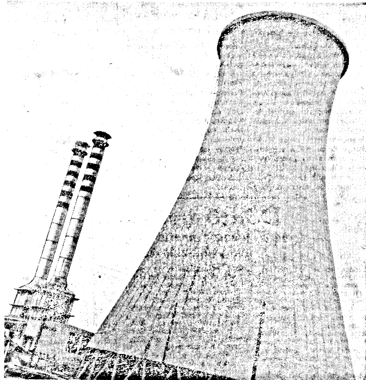
Ime az aradi villanygyár új, negyvennyolc méter magas, 2500 köbméter víz lehűtésére alkalmas impozáns, korszerű hűtőtornya
