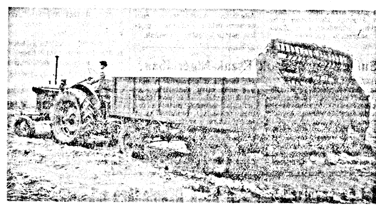
Az ötvenesi állami gazdaság nagy kiterjedésű földjeire a tavaszi vetés megkezdése előtt jó, érett trágyát szórnak. Az utánfutóra szerelt emés szerkezet segítségével kiküszöböltek a trágya szétterítésénél eddig alkalmazott fizikai munkát.
