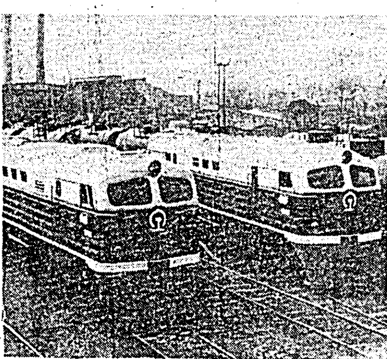
R. P. CHINEZĂ. — La uzina de locomotive din Talian se construiesc aceste locomotive Diesel cu o putere de tracțiune de 2000 C.P.
