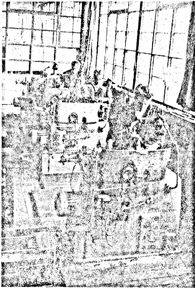
A Victoria óragyárban korszerű önműködő esztergagépeken készítenek a különböző nagy pontosságot igénylő alkatrészeket. E gépeken egyszerre több műveletet is elvégeznek s ezzel lényegesen növelik a munka termelékenységét.
