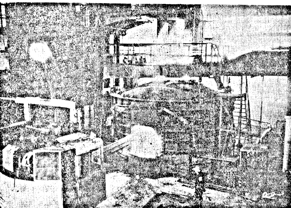
SZOVJETUNIO. Cseljabinszk legnagyobb nehézipari üzemében nagy befogadóképességű villamos kemence kezdte meg működését. E villamos kemence üzembehelyezésével befejezést nyert ennek az új ipari létesítménynek építése. Képünk az üzembehelyezési villamos kemencét ábrázolja.
