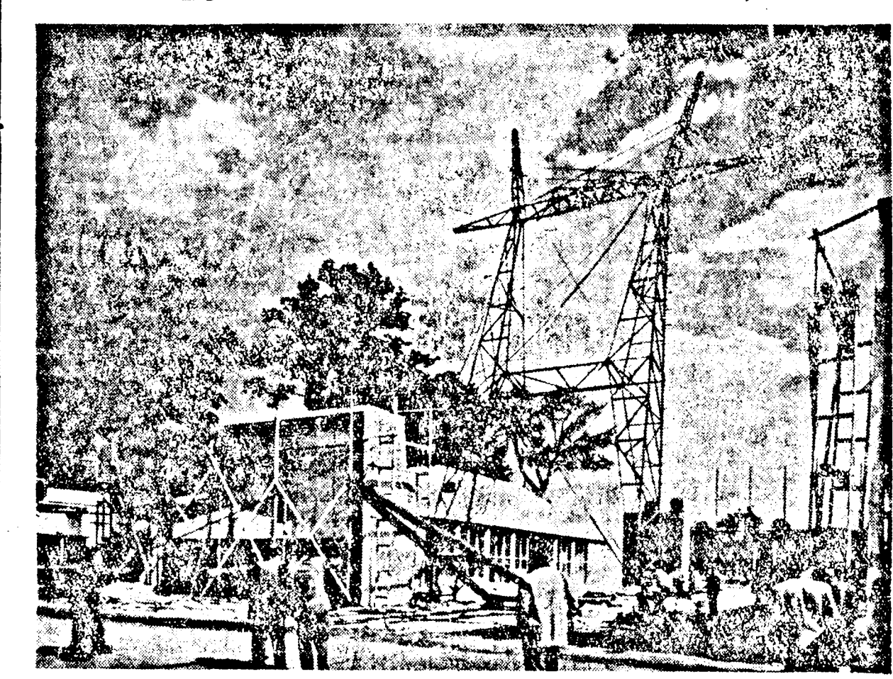
A Magyar Népköztársaságban elkészítették a 120 Kilowattos villamosvezeték számára alkalmas új típusú tartóoszlop tervét. Az új típusú tartóoszlop majdnem ezer kilóval könnyebb, mint a régi. A magyar iparnak ezt az új készítményt bemutatják majd a budapesti ipari vásáron. Képünkön: az új tartóoszlop.
