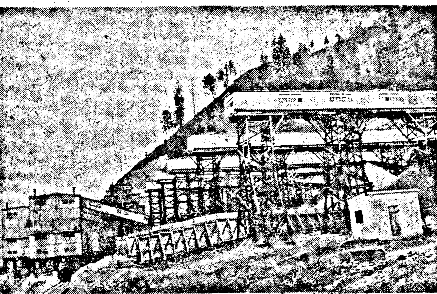
A duzzasztó gát kiépítéséhez szükséges beton előállítására épült a békási betongyár. Az önműködő gyár naponta 4000 köbméter beton termelésére alkalmas. A képen a betongyár látható.
