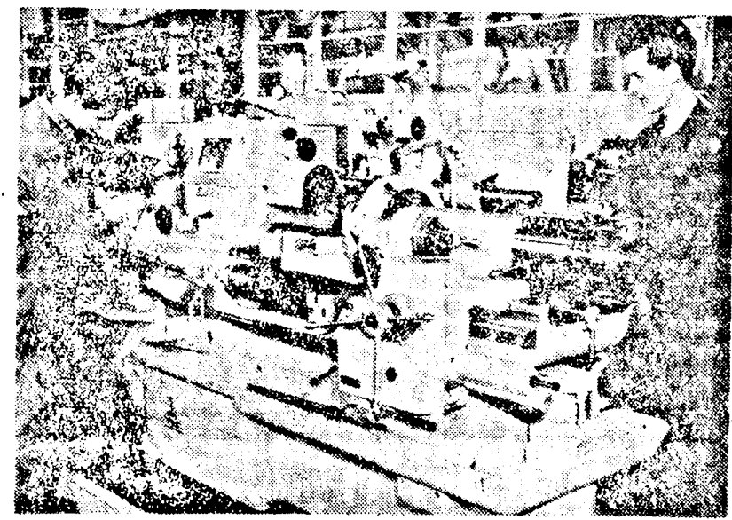
A gottwaldovi (Csehszlovák SzK) tñommechanikai vál- lalatban nagy pontosságú szerszámgepek készülnek az RNK számára. Ezek között szerepel a képen látható pneumatikus befogófejjel ellátott reverver pad.
