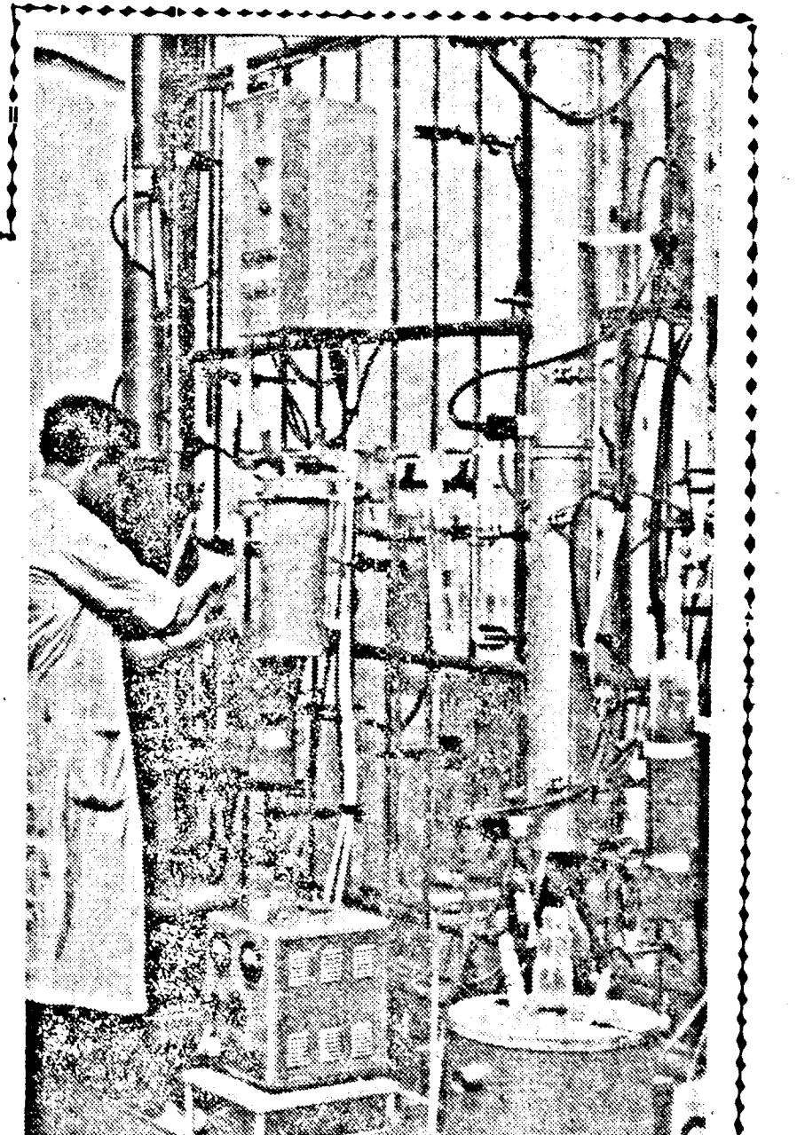
Freiberg mellett, Muldenhüttenben (NDK) nem mindennapi intézet működik, mely a nyom-elemek előállításával foglalkozik. Képünkön a rádióaktív germánium előállítására szolgáló hatalmas desztillációs oszlopok láthatók.
