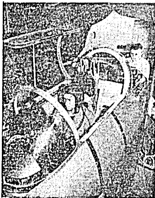
În RS Cehoslovacă, a fost construit un aparat special pentru pregătirea piloților de avioane supersonice. În clișeu: aspect din timpul funcționării unui astfel de aparat.
