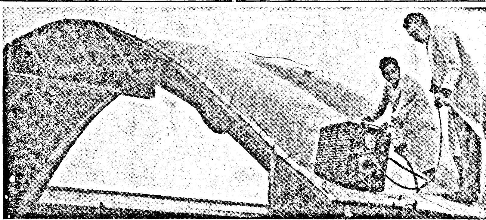
A fővárosi Építészeti és Építkezés-Gazdasági Kutatóintézet az új eljárásokkal és az új építőanyagok — egyszerű és vasbeton, előkészített betonszerkezetek — hatékonyságának kikísérletezésével foglalkozik. Képünkön: ultrahang segítségével ellenőrzik egy új típusú tetőburkolat betonanyagának szilárdságát.
