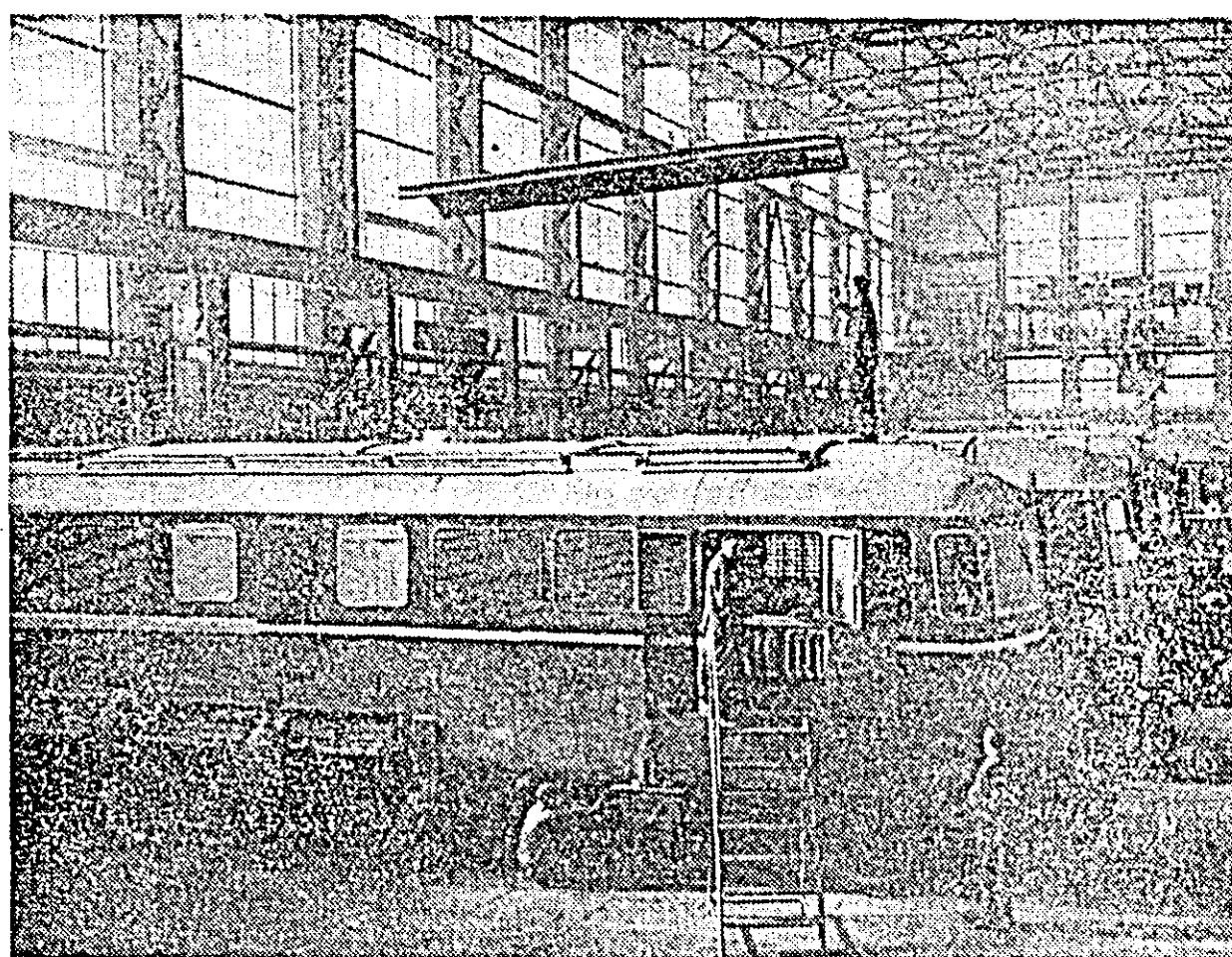
La fabrica de locomotive Diesel, din cadrul uzinei „Electroputere” din Craiova se va termina în curînd construcția celei de a 100-a locomotive electrice românești. ÎN CLISEU: aspect din hala de montaj a fabricii de locomotive Diesel de la uzina „Electroputere” Craiova.
